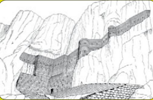
שרטוט: איור. ליון רטמיאר לפי צבי אילן שחזור חזית המצודה העותמאנית.
