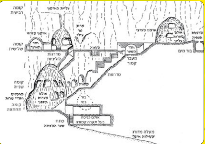
שרטוט: ליון רטמיאר לפי אברהם איזנברג ואמנון קדרון חקר פנים של המצודה העותמאנית.
